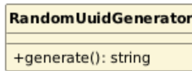
Figura 84: Classe — RandomUuidGenerator
