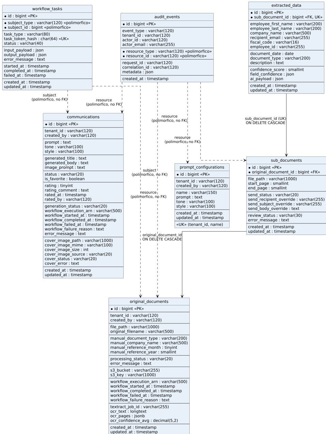
Figura 123: Schema Relazionale
