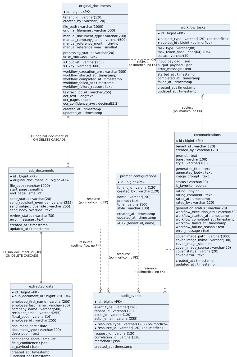
Figura 124: Schema ERD
