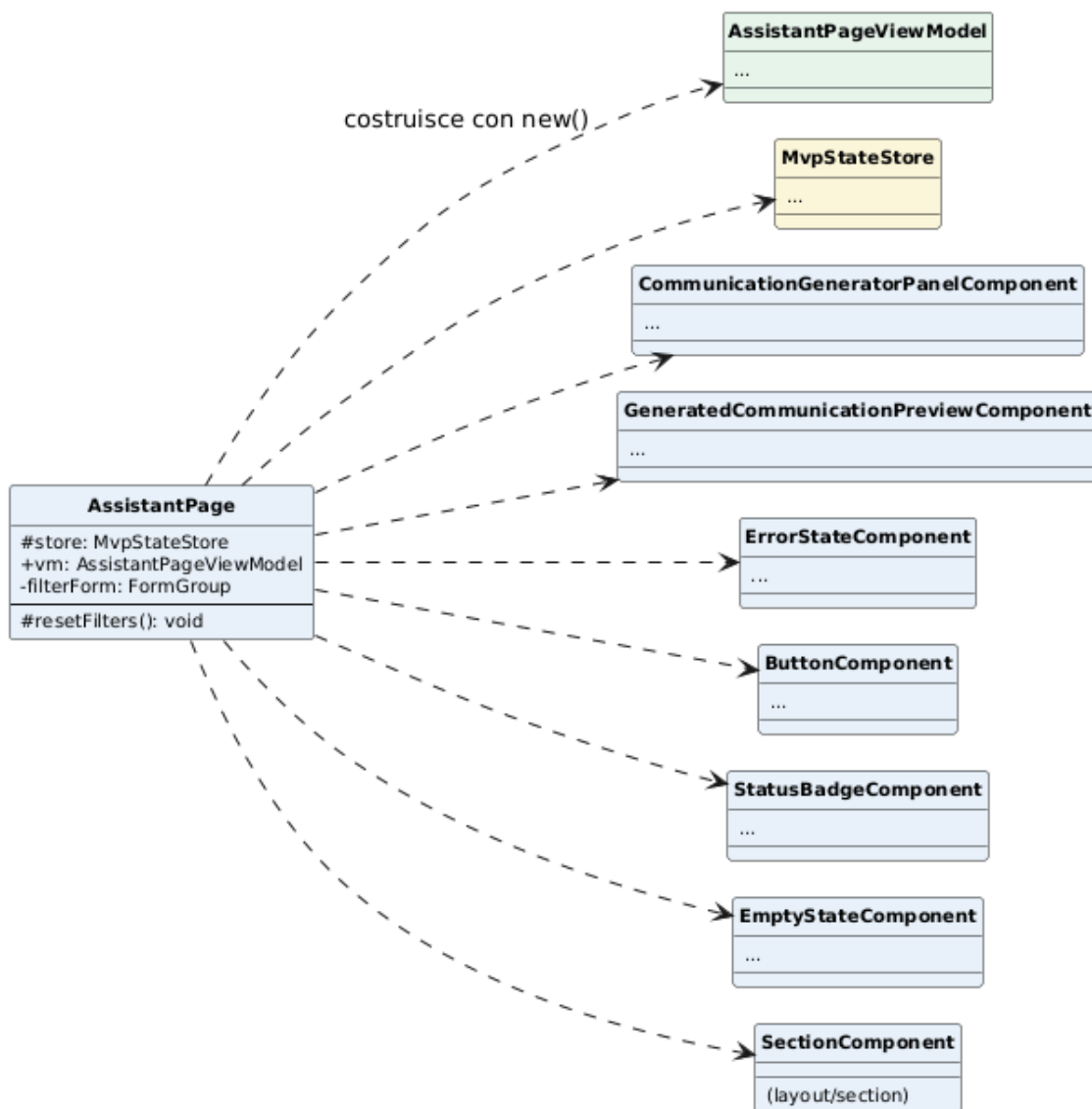
Figura 119: Classe — AssistantPage
