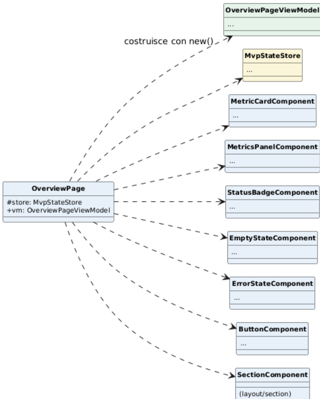
Figura 121: Classe — OverviewPage
