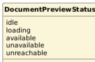
Figura 107: Tipo — DocumentPreviewStatus
