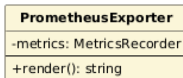
Figura 88: Classe — PrometheusExporter
