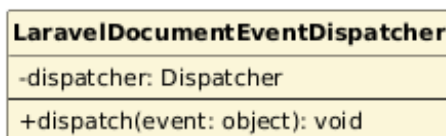
Figura 38: Classe — LaravelDocumentEventDispatcher
