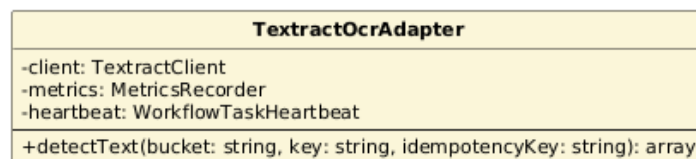
Figura 34: Classe — TextractOcrAdapter
