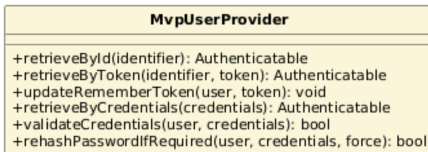
Figura 82: Classe — MvpUserProvider
