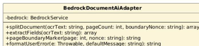
Figura 35: Classe — BedrockDocumentAiAdapter
